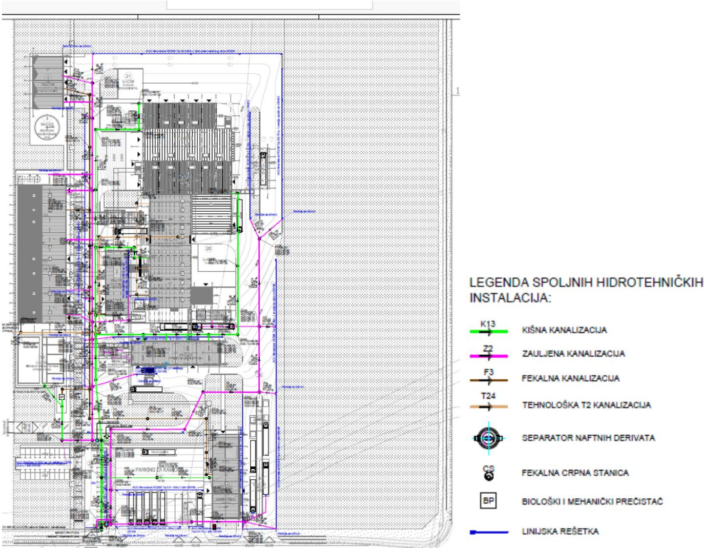
Imagina 9.5 Situația instalațiilor hidrotehnice de canalizare
