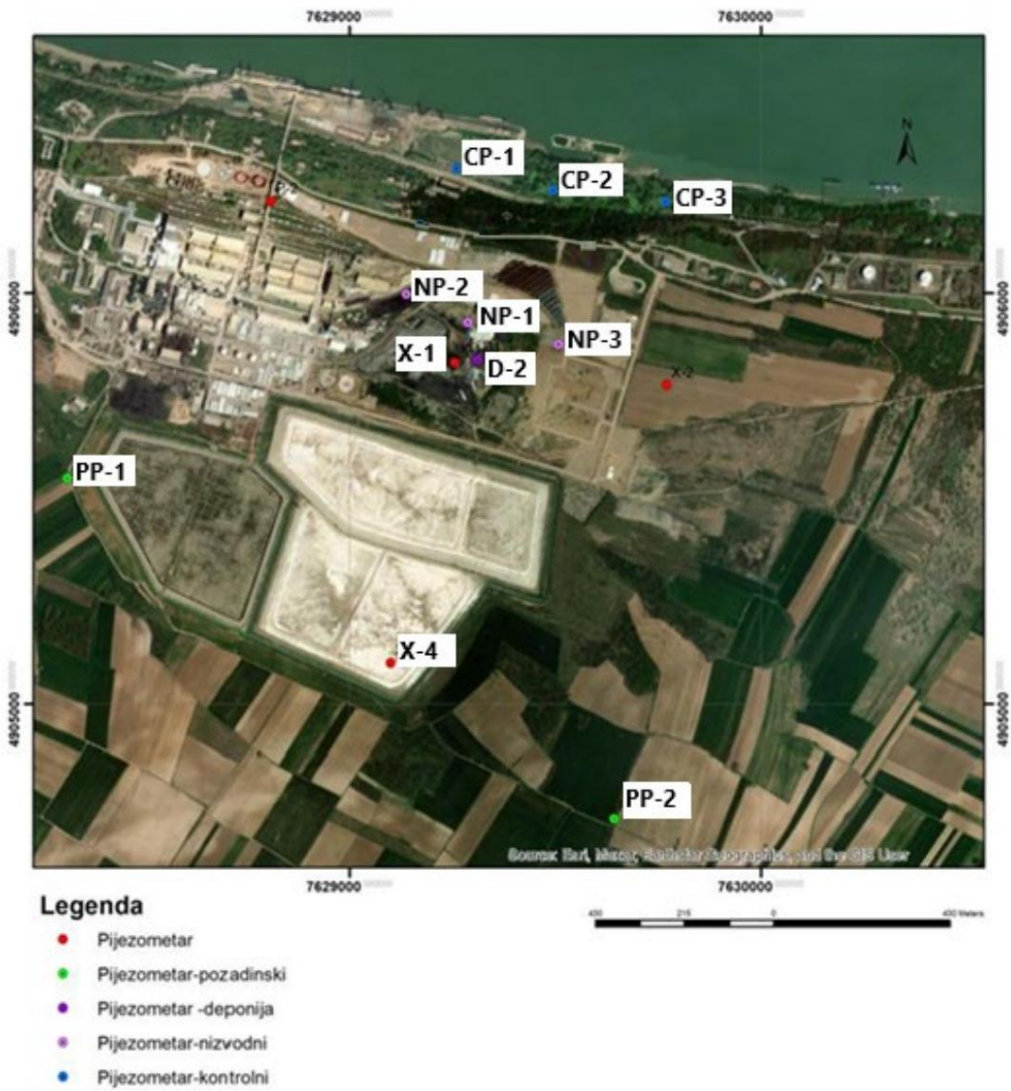
Imaginea 9.7.2 Propunere de cadru pentru amenajarea piezometrelor pentru monitorizare
